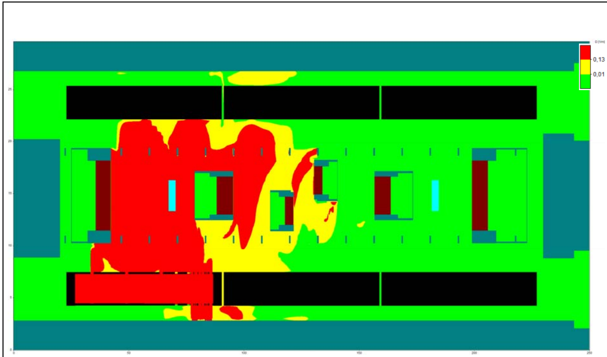
Bild 5: Optische Dichte pro Weglänge in einer Höhe von ca. 1,5 m über der Bahnsteigoberkante 30 Minuten nach Brandbeginn (Grundriss)
