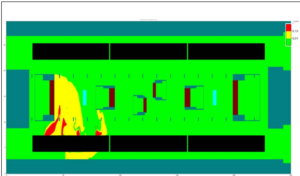
Bild 3: Optische Dichte pro Weglänge in einer Höhe von ca. 2,5 m über der Bahnsteigoberkante 9 Minuten nach Brandbeginn (Grundriss)
