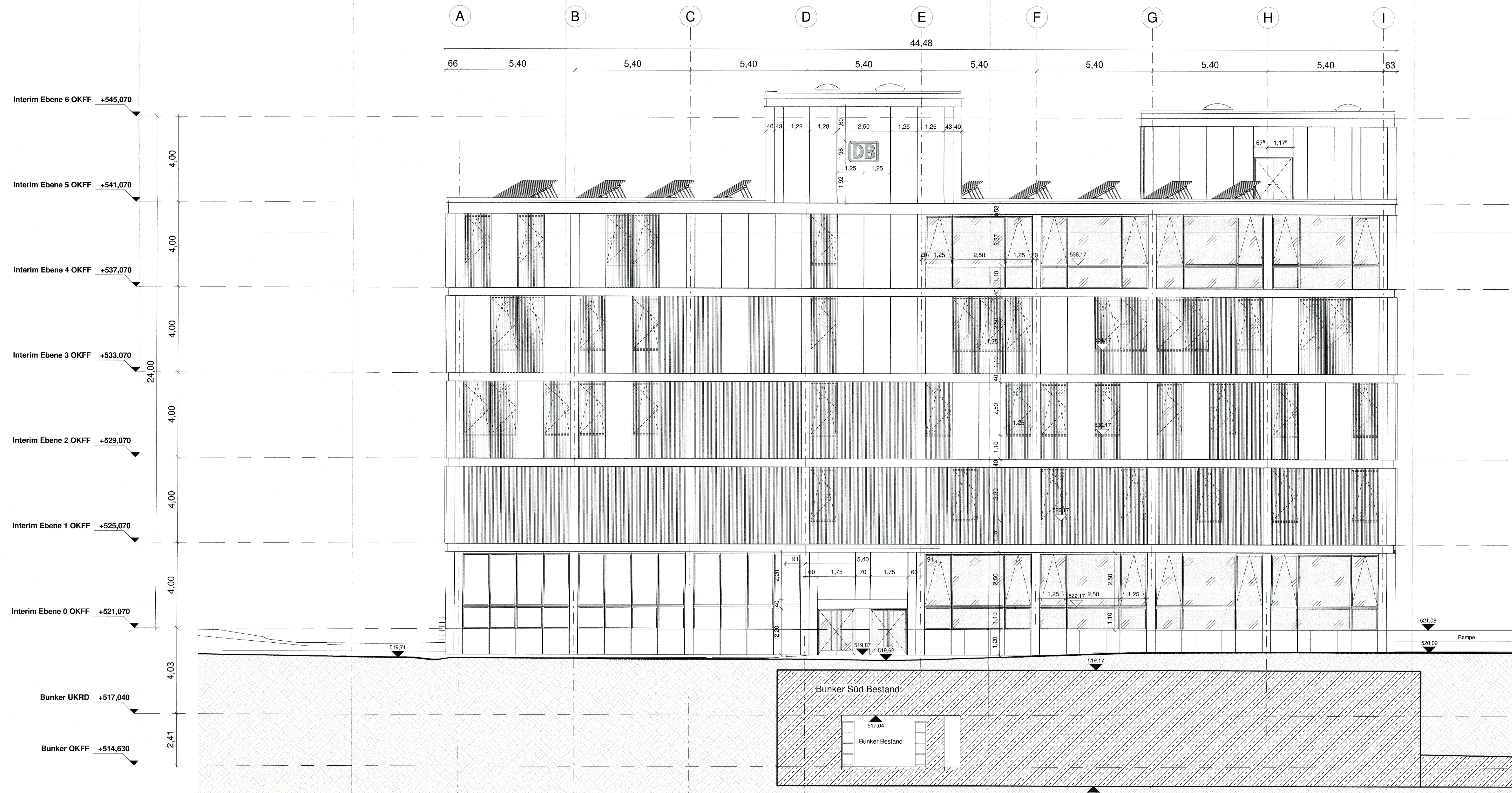
Ansicht Süd 1:100
